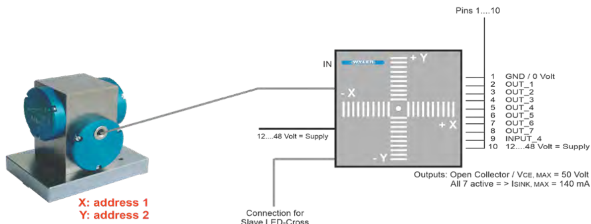
Zwei ZEROTRONIC-Sensoren Montage- Vorrichtung und einem Anschluss
