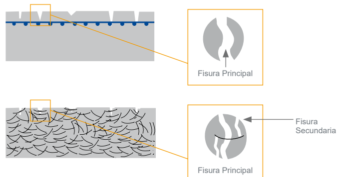
Refuerzo Convencional
