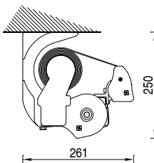
Montaje a techo con soporte pared/techo
