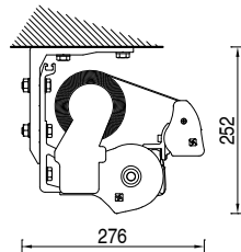
Montaje a techo
