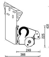
Montaje entraparedes
