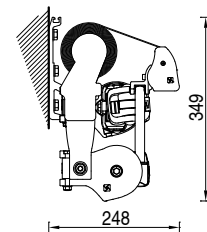
Montaje con brazos cruzados
