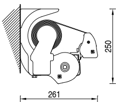
Montaje a pared con soporte pared / techo
