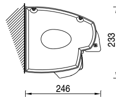
Montaje con tejadillo
