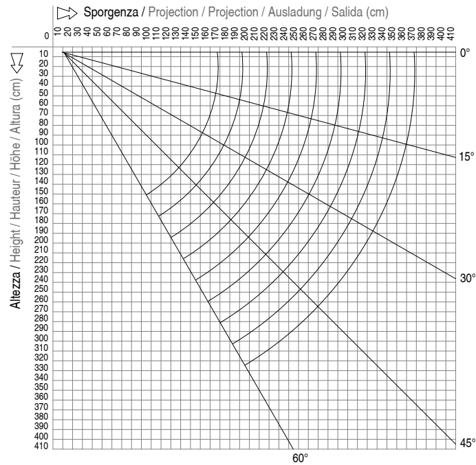
Diagrama de proyección - Montaje a pared / techo
