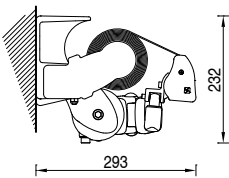
Montaje a pared
