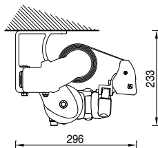
Montaje a techo con soporte extruido
