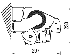
Montaje a pared con soporte extruido
