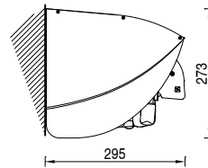
Montaje con tejadillo
