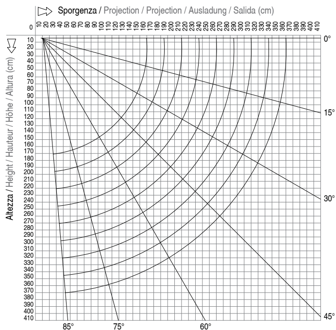
Diagrama de proyección - Montaje a pared/techo
