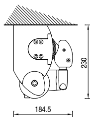
Montaje a techo
