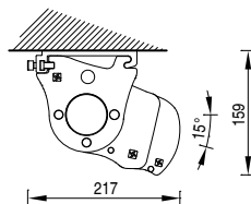
Montaje a techo 15°
