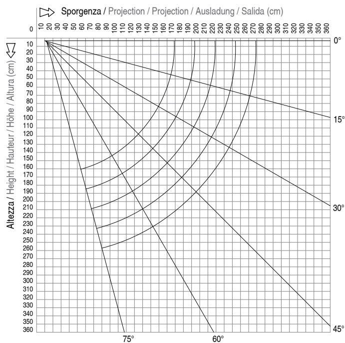
Diagrama de proyección - Montaje a pared
