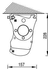
Montaje a techo 90°
