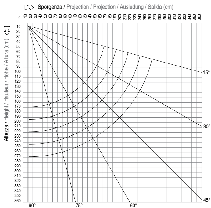
Diagrama de proyección - Montaje a techo
