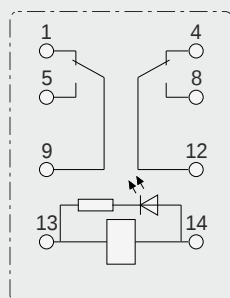
2C con indicador
