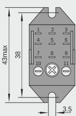
3C, montaje frontal (fijación superior)
