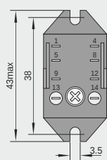
2C, montaje frontal (fijación superior)
