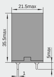
Circuito impreso, 2C
