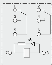
Conexiones internas, con indicador (vista inferior)
