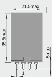
Circuito impreso, 4C
