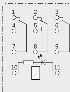
3C con indicador
