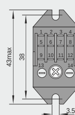
4C, montaje frontal (fijación superior)
