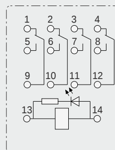
4C con indicador
