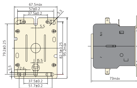
NCK3-25~40
