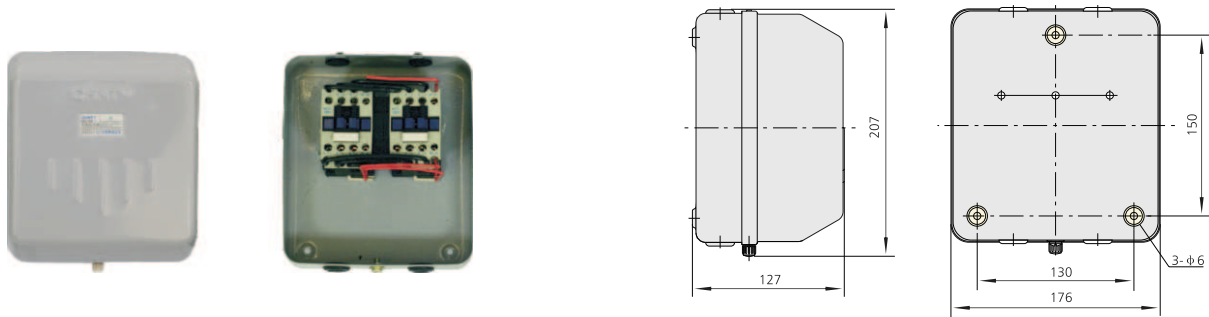
NQ2-15NB
