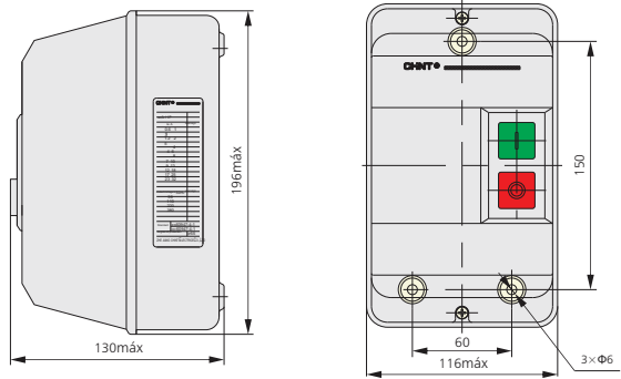
NQ3-11P
