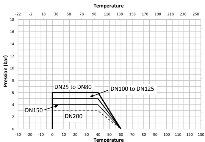
PVC-U
