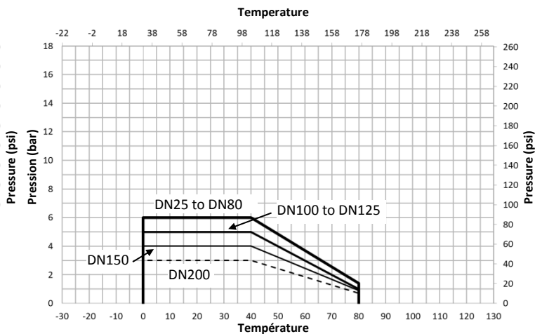
PVC-C
