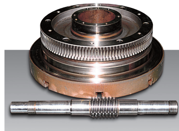
Sistema de husillo / corona después de 7 años de uso
