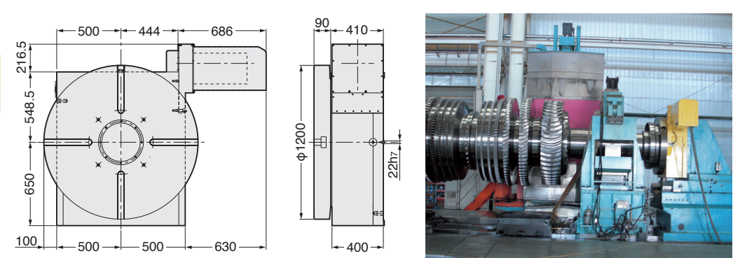
Indexación del eje de la turbina.
