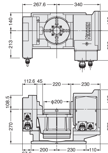
5AX-DD200B
