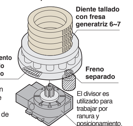
CNC1800 y estructura de apoyo Indexación / sujeción del anillo de la turbina
