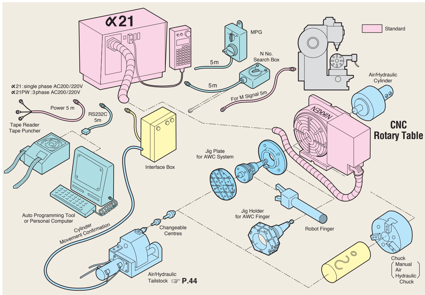
CONTROL \alpha 21 para amplia capacidad
