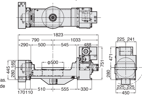
Combinación de CNC503H & CNC302T
