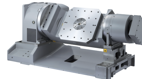
5AX-500 con placa cuadrada
