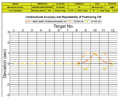
Precisión unidireccional y repetibilidad de posicionamiento
