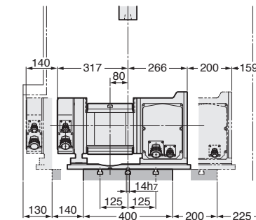
5AX-DD200
