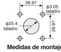
Medidas de montaje
