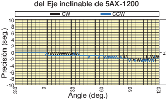
Medición de precisión del eje inclinado \pm 3 sec.
