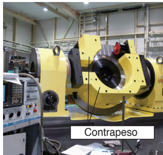
Precisión de medición del eje rotativo \pm 3 sec.
