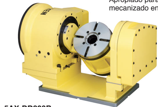
5AX-DD200B
