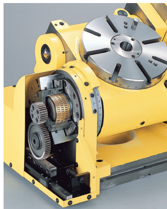
Potente sistema de freno
