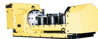
Tres set de platos hidráulicos usados para el amarre de la pieza
