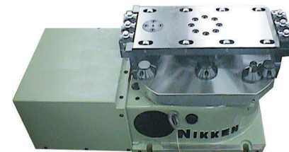
Pallet con unidad de bloque y acoplador automático.
