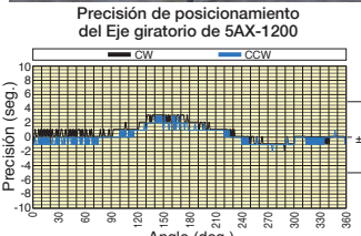
Precisión de medición del eje rotativo \pm 3 sec.
