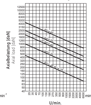
Axialbelastung Lebensdauer des Wälzlagers: 2000 Std. Axial load Service life of roller bearing: 2000 h
