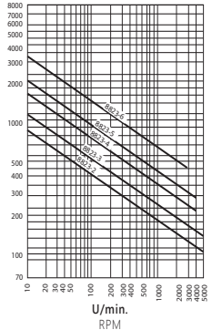
Axialbelastung Lebensdauer des Wälzlagers: 2000 Std. Axial load Service life of roller bearing: 2000 h
