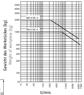
Radialbelastung Lebensdauer des Wälzlagers: 2000 Std. Radial load Service life of roller bearing: 2000 h
