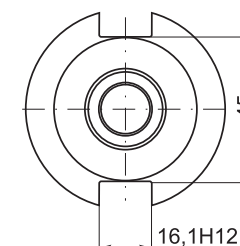
DIN 2080-40
