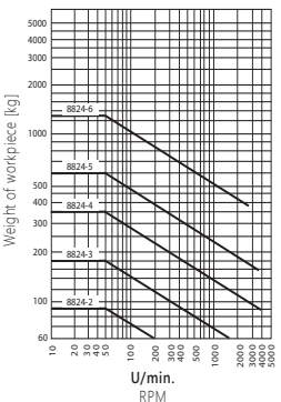
Radialbelastung Lebensdauer des Wälzlagers: 2000 Std. Radial load Service life of roller bearing: 2000 h
