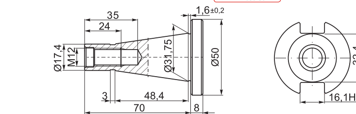
DIN 2080-30
