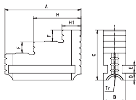
Garras duras monoblock
