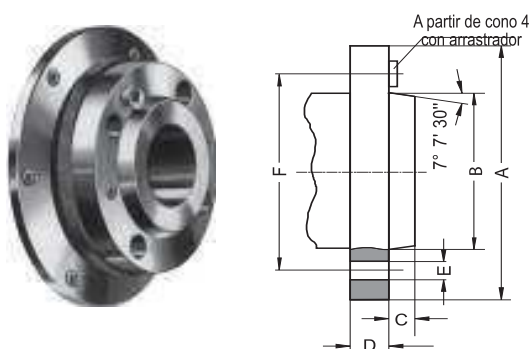
DIN 55027 & ISO 702/III
