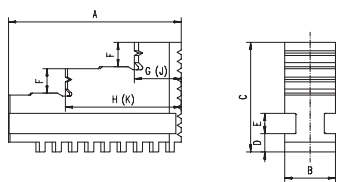
Garras duras monoblock interiores y exteriores
