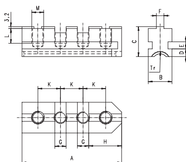
Garras duras base
