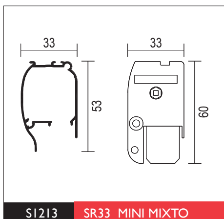
Testero Mini SR33 End cap Mini SR33 Embout Mini SR33 Kassettenkappe Mini SR33
