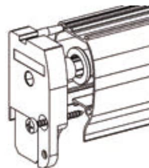
Testero con tornillo de sujeción al cajón Fixing of end cap at the box Embout fixé au caisson par vis Befestigung Kassettenkappe an der Kassette
