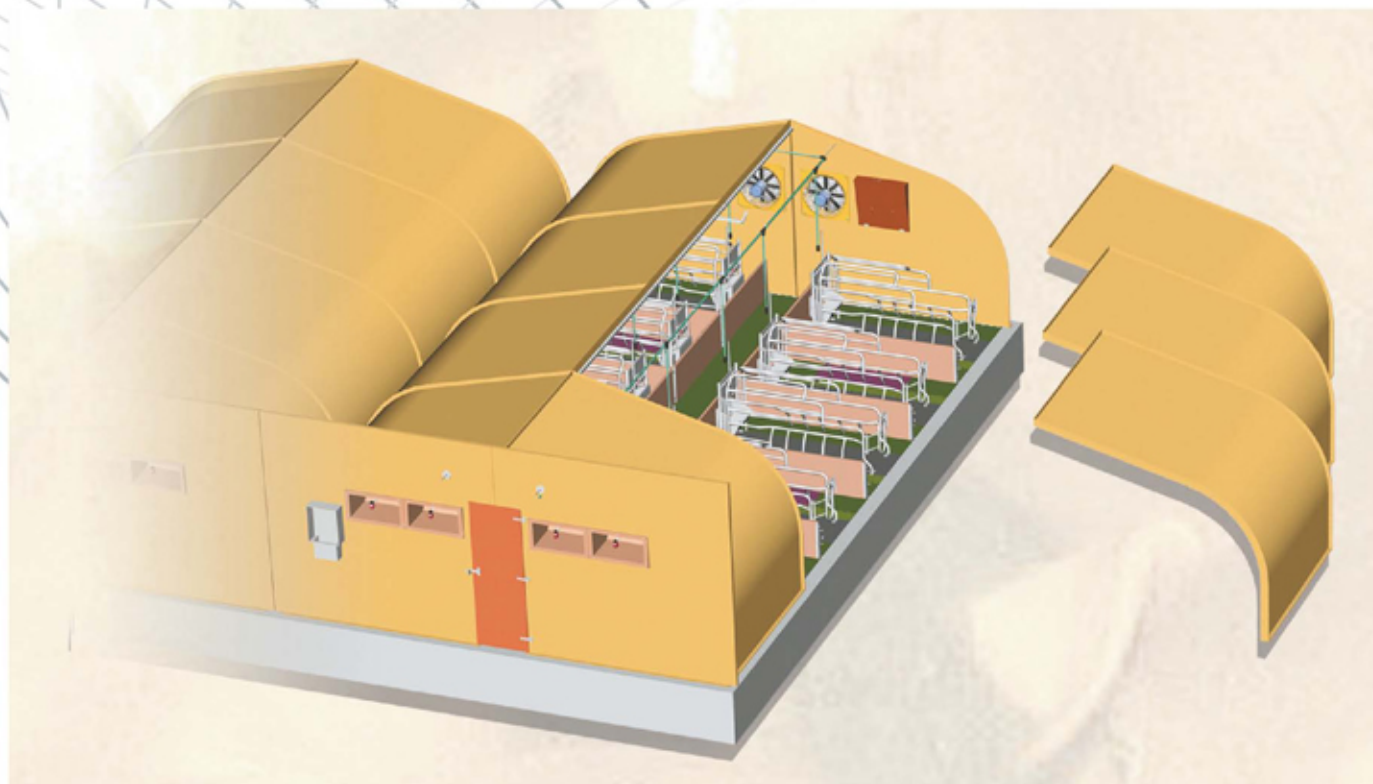
Nave Modular Módulos de 5,60m de ancho longitud variable según necesidades de capacidad. Longitudes desde 4,80m, 7,20m, 9,60m, 12,00m, 14,40m ..... 24,00m, etc.....
