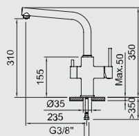
62019 (61428 + 61237) PURE + Fregadero Chef 3 vías PURE + 3 ways sink mixer PURE + Mitigeur évier 3 voies PURE + Torneira Chef 3 vías
