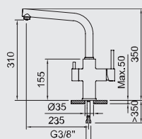
61429 (61428 + 61102) PURE + Fregadero Chef 3 vías PURE + 3 ways sink mixer PURE + Mitigeur évier 3 voies PURE + Torneira Chef 3 vías
