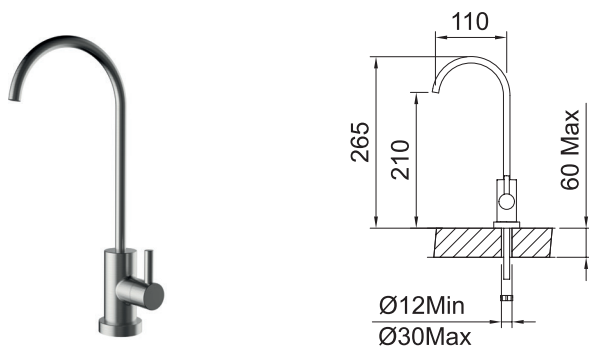
61480 Grifería agua filtrada Water quality sink Robinet avec sortie eau purifiée Torneira para água filtrada
