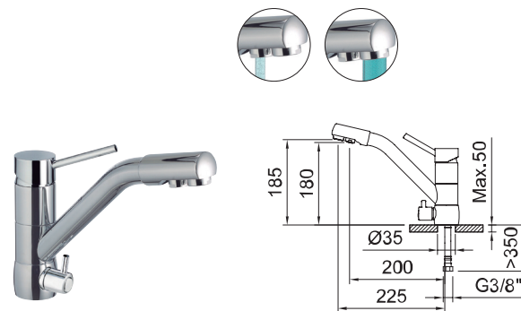
98760 Grifo de cocina 3 vías 3 Way sink mixer Mitigeur évier à 3 voies Torneira de banca de 3 vías
