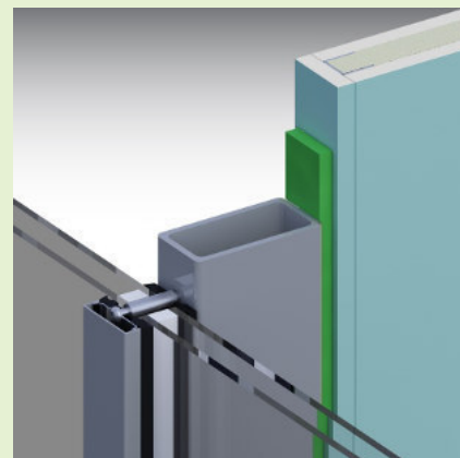
TP600 Espuma impregnada illmod
