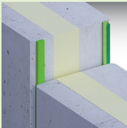
SP522 Sellador híbrido para fachada FA870 Silicona para piedra natural PR102 Fondo de junta (interior) TP600 Espuma impregnada illmod (ext.)
