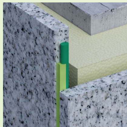
SP522 Sellador híbrido para fachada PR102 Fondo de junta
