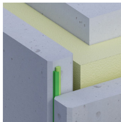
SP522 Sellador híbrido para fachada FA870 Silicona para piedra natural PR102 Fondo de junta
