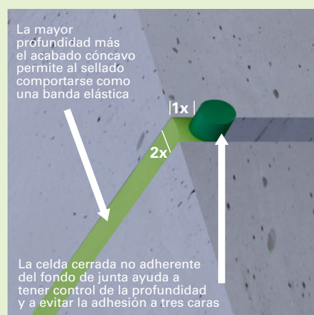
Junta de control en muro de hormigón
