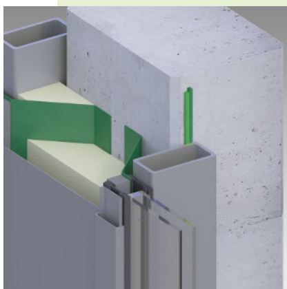
TP600 Espuma impregnada illmod ME220 Membrana EPDM exterior
