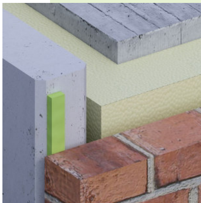
TP600 Espuma impregnada illmod
