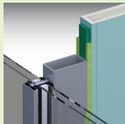
FA101 Silicona neutra para cerramientos FS125 Silicona para ventanas y fachadas LD704 Sellador acrílico PR102 Fondo de juntas
