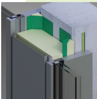
FA101 Silicona neutra para cerramientos FS125 Silicona para ventanas y fachadas PR102 Fondo de juntas ME220 Membrana EPDM exterior
