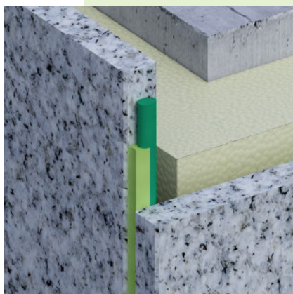
FA870 Silicona para piedra natural PR102 Fondo de junta
