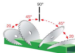
Diagramma di taglio Cutting diagram/Diagramme de coupe Diagrama de corte/Schnitttdiagram
