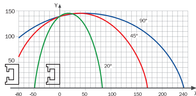
Diagramma di taglio Cutting diagram/Diagramme de coupe Diagrama de corte/Schnitttidiagram
