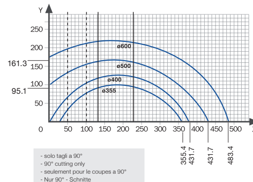
Diagramma di taglio Cutting diagram/Diagramme de coupe Diagrama de corte/Schnittdiagram
