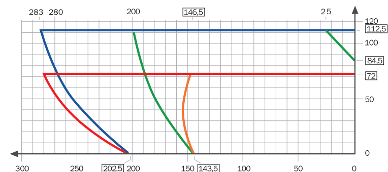
Diagramma di taglio Cutting diagram Diagramme de coupe Diagrama de corte/Schnittdiagram
