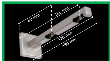
Soporte Doble Pared
