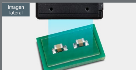
Corrección de posición 3D con LJ-X8000SO(55209)
