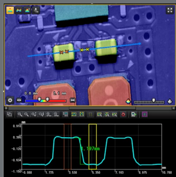
Corrección de posición 3D con LJ-X8000SO(55209)
