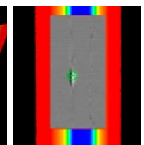
Imagen después de extraer la altura + el daño
