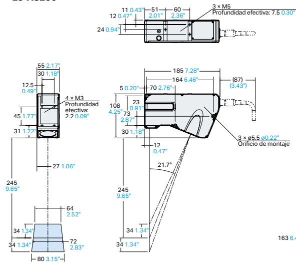
LJ-X8200
