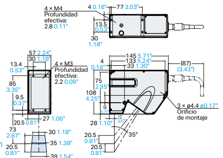
LJ-X8080
