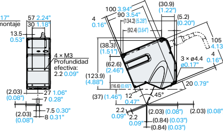
LJ-X8020 en configuración de reflexión especular
