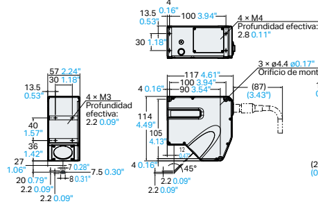
LJ-X8020
