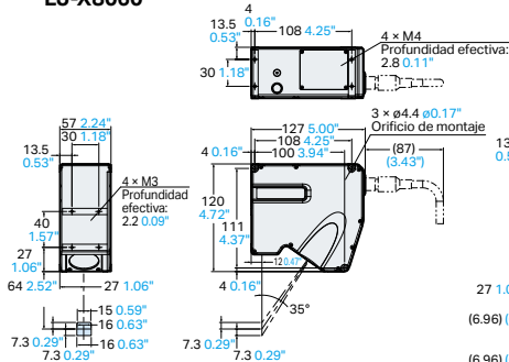
LJ-X8060
