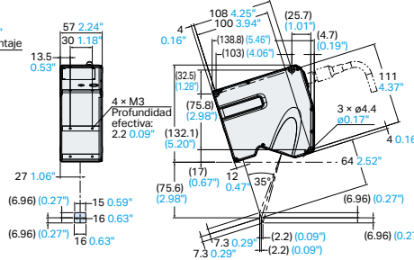
LJ-X8060 en configuración de reflexión especular
