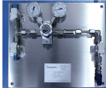
Panels de regulación
