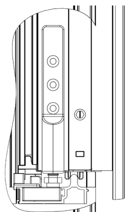
Posición abierta
