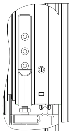
Posición cerrada
