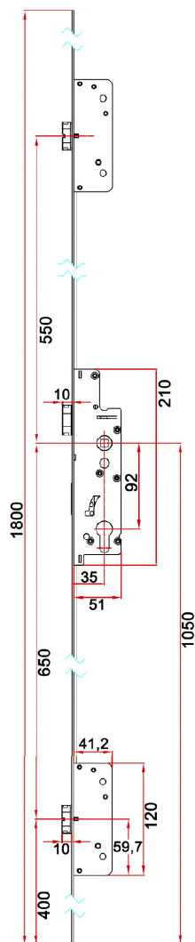
POSICIÓN ABIERTA
