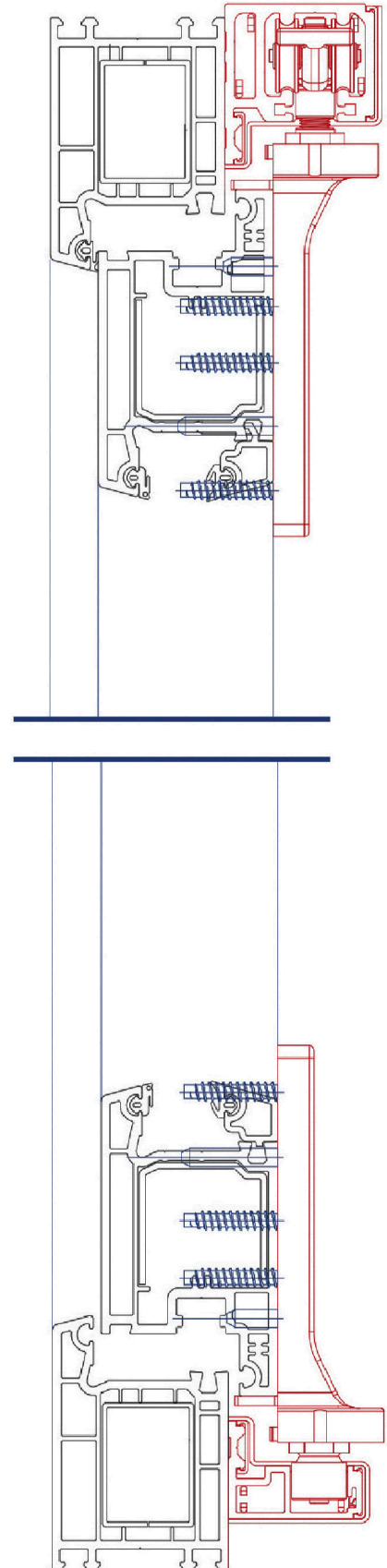
Versión corredera superior (hasta 80kg)
