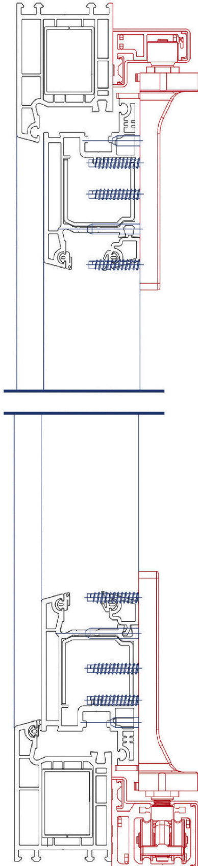
Versión corredera inferior (hasta 100kg)
