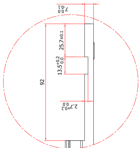
DETALLE Y ESCALA: 5/1
