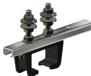
Par de estribos soporte para SMGX incl. perfil de soportación
