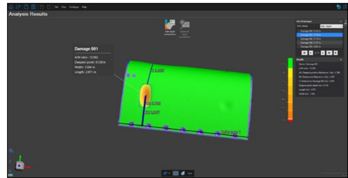
Abolladuras en el borde principal del ala de un avión medidas con VXintegrity / SmartDENT 3D
