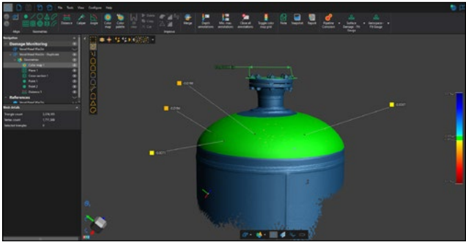
Control dimensional de rebordes y corrosión puntual medida en la cabeza de un recipiente a presión con VXintegrity / Supervisión de daños
