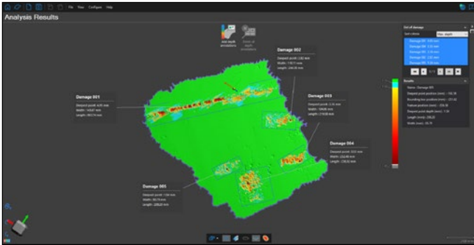
Corrosión en el piso de un tanque analizada con VXintegrity / Daños en la superficie
