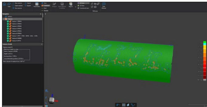
Daño por corrosión en una tubería analizado con VXintegrity/Pipecheck
