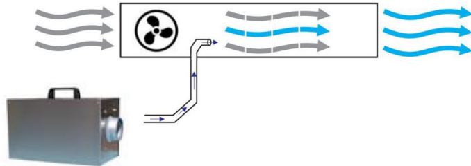
Sistema de inyección directa en conducto
