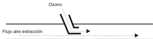
Sistema de inyección directa en conducto
