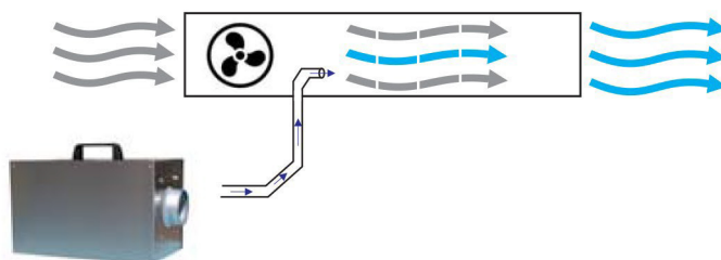
Sistema de inyección directa en conducto
