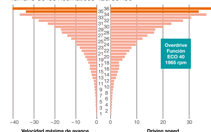
Serie M4003. Transmisión “Dual Speed” (36/36) Tamaño de los neumáticos 420/85R30
