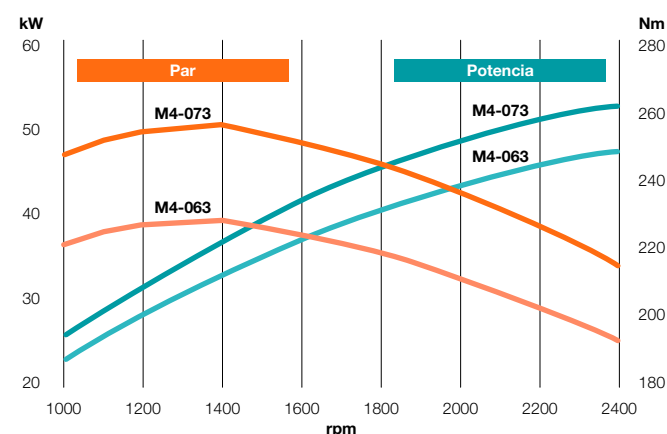
Potencia y par
