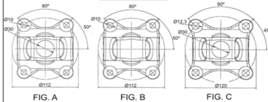
TIPOS DE BRIDA
