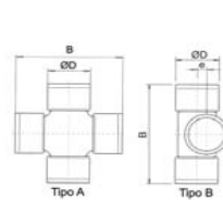
TIPO DE CRUZ
