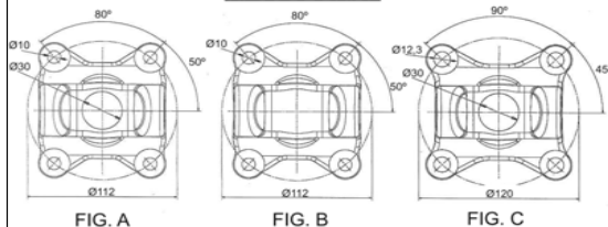
TIPOS DE BRIDA
