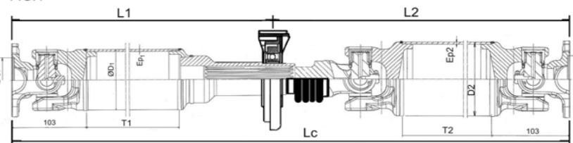
FIG.4 CARDAN 2 TRAMOS
