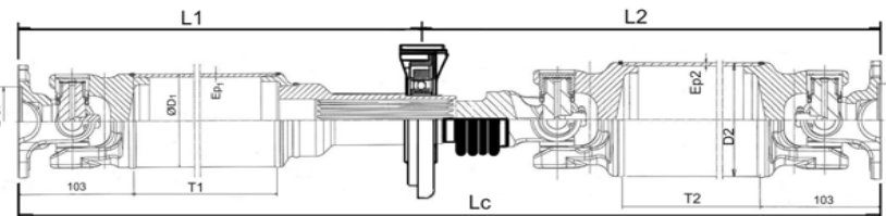
FIG.4 CARDAN 2 TRAMOS
