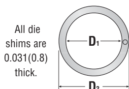
114/MARATHON® DIE SHIM PACKAGE
