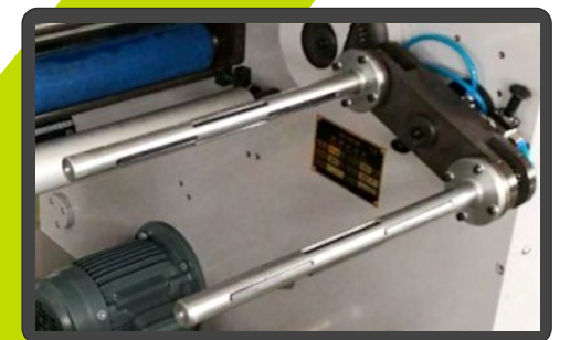
Rebobinador doble para cambio rápido
