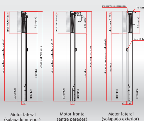
Motor lateral (solapado interior)
