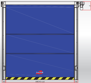
Motor frontal (semitunel)
