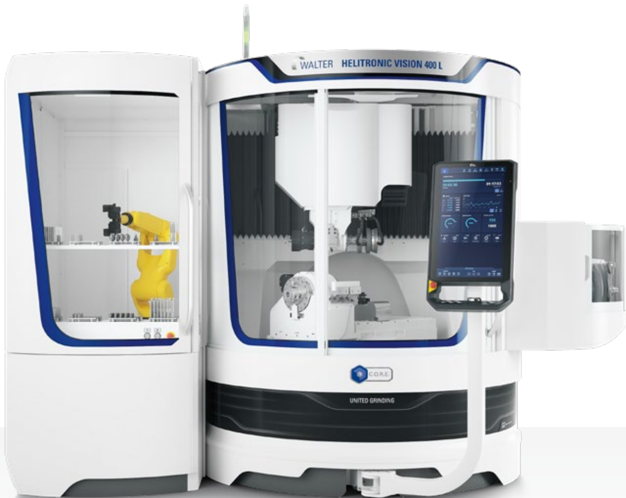
HELITRONIC VISION 400 L mit den Optionen Scheibenwechsler (rechts) und Robotlader (links)
