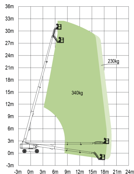
Curva de amplitud de plataforma ZT30J
