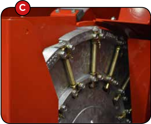
C. Disco dosificador con pinzas
