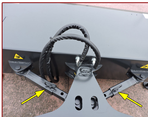
▲ Angulación lateral regulable mecánicamente (izquierda - derecha). Mechanically adjustable lateral angulation (left-right).
