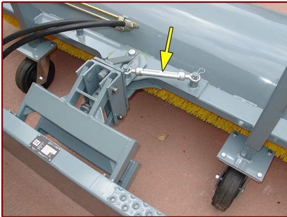
▲ Angulación lateral regulable mecánicamente izquierda - derecha (hidráulica opcional) Mechanically adjustable lateral angulation left-right (optional hydraulic)
