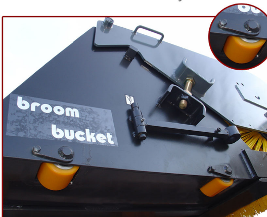
▲ Ruedas deslizamiento cuchara - option Wheels for sliding the bucket - option
