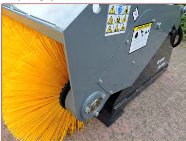
▲ Sistema regulación cepillo central en el interior. Adjusting system for the central brush inside.
