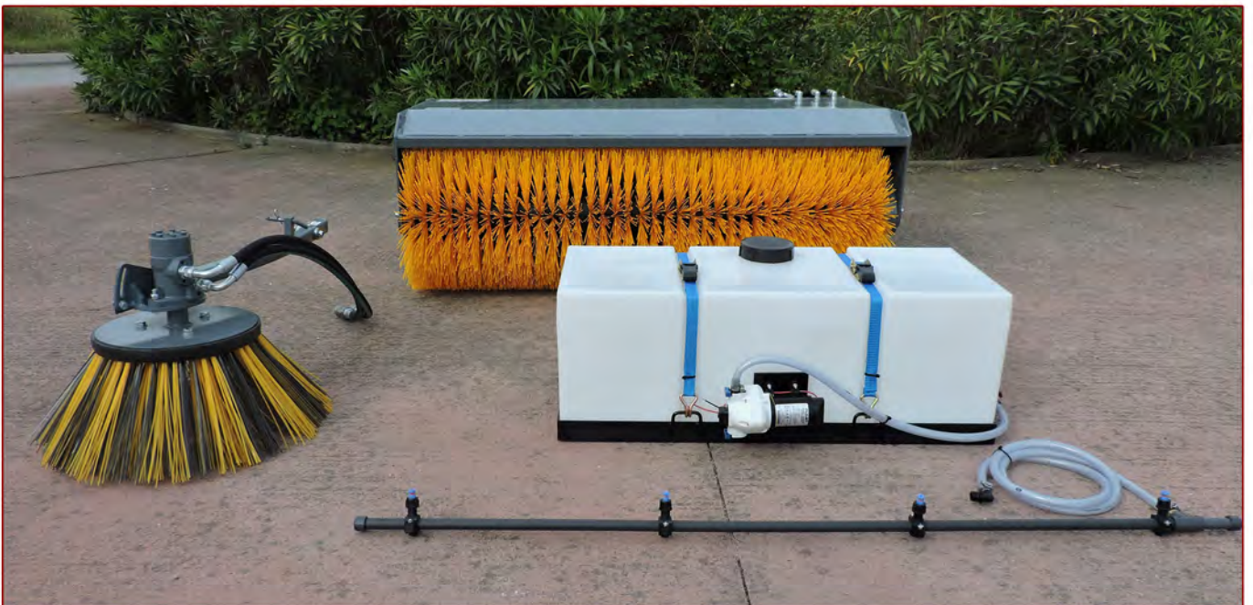
▲ Sistema de cepillo lateral y sistema de riego con soporte de depósito - opción Side sweeper system and sprinkler system with tank support - option
