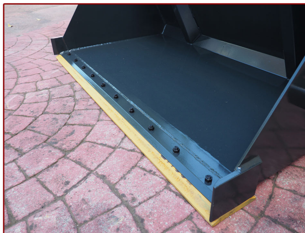
▲ Cuchilla atornillada doble uso más otra soldada Bolted blade of dual-use and other welded
