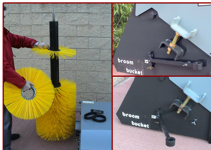
▲ Sistema para facilitar el cambio del cepillo central - opción System for changing the central brush in a easier way - option
