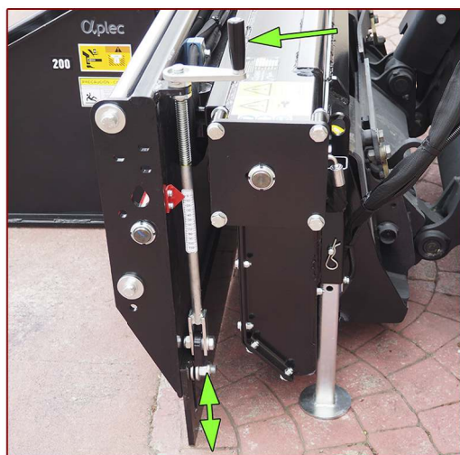
▲ Ajuste mecánico, independiente derecha-izquierda, para regular el espesor de la capa del material a extender (eléctrico opcional). Mechanical adjustment, independent right-left, to regulate the layer thickness of the material to be extended (optional electric).
