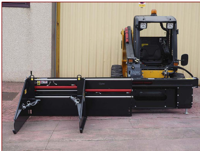
▲ Desplazamiento lateral hidráulico. Hydraulic side shift.
