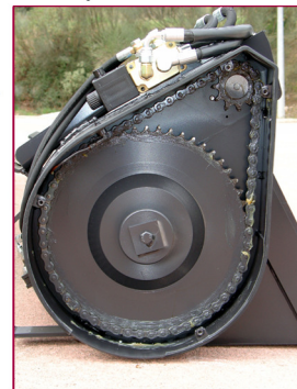
▲ Transmisión por cadena Chaine transmission
