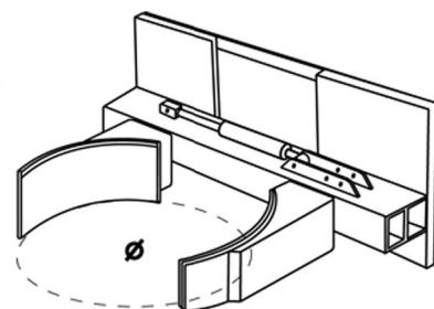
▲ Fijaciones culata cilindro para el ajuste de la apertura-cierre de las mordazas Cylinder head fixings for adjusting the opening-closing of the jaws
