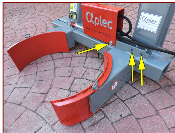
▲ Fijaciones culata cilindro para el ajuste de la apertura-cierre de las mordazas Cylinder head fixings for adjusting the opening-closing of the jaws
