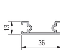
AP-G1 Nº de artículo 209596 (Longitud máx. 6 m)
