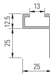
AP-5-F1 Nº de artículo 311759 (Longitud máx. 6 m)
