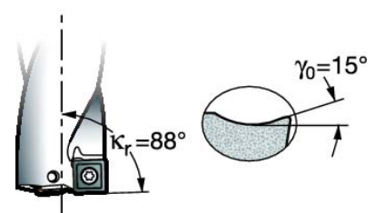
CoroDrill® 880
