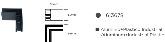
Esquina horizontal de montaje en superficie/Surface Mounted Horizontal Corner
