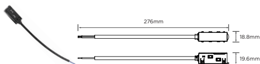
Paquete de accesories para montaje de Suspensión/Front Conductive Module
