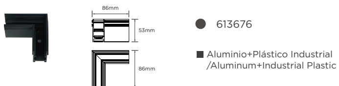
Esquina horizontal empotrada/Recessed Horizontal Corner
