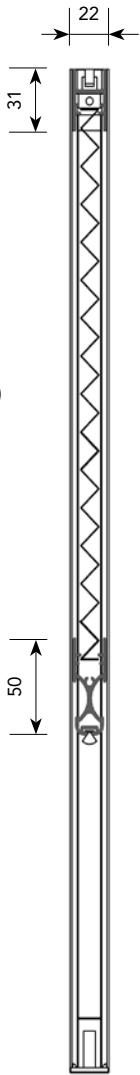
SECCIÓN VERTICAL (mm) Section verticale (mm) Secção vertical (mm)
