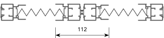
2 HOJAS CON CIERRE CENTRAL 2 vantaux avec fermeture centrale 2 folhas com fecho central
