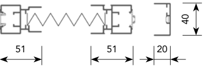
1 HOJA / 1 vantail / 1 folha
