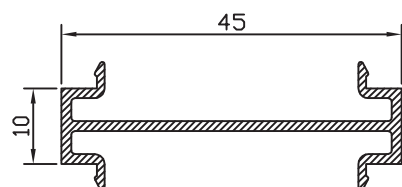
UNIÓN CARPINTERIA 22003
