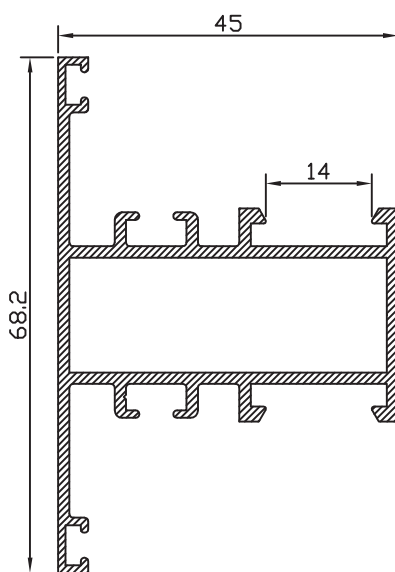
PILASTRA 22580
