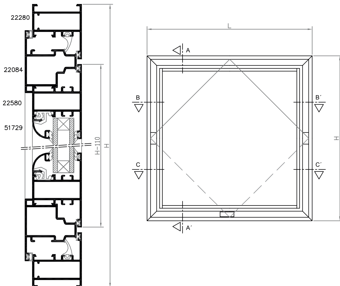
SECCIÓN A-A'
