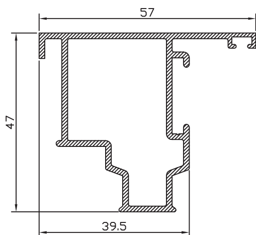
PERFIL PIVOTANTE 22084
