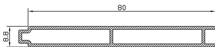
LAMA PORTICONES 60676
