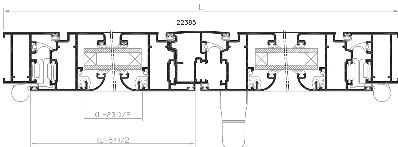
SECCIÓN B-B'
