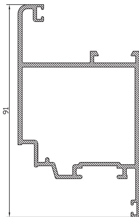
HOJA CAM. 40 PUERTA 23389
