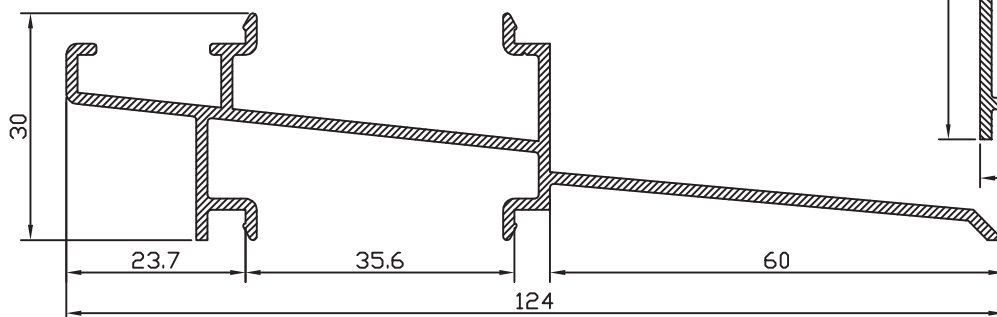
CONDENSACIÓN PALA DE 60 22239
