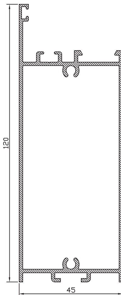
ZÓCALO MARCO PUERTA 23476
