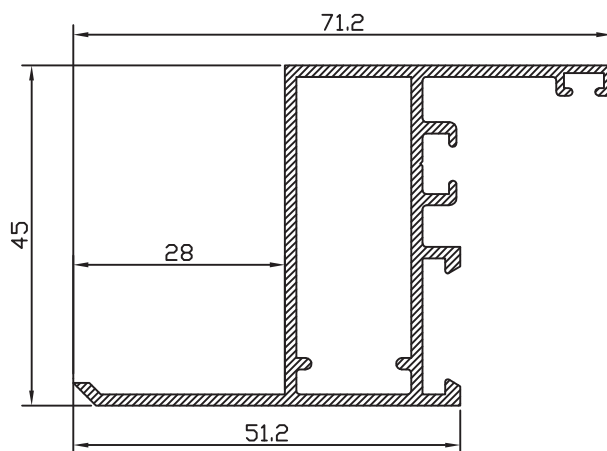
MARCO CON PREMARCO 22281
