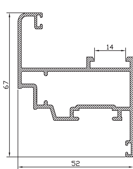
HOJA VENTANA 22388
