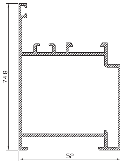
MARCO C/40 ENRAS. PUERTA 23282
