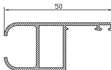
HOJA CONTRAVENTANA 22393
