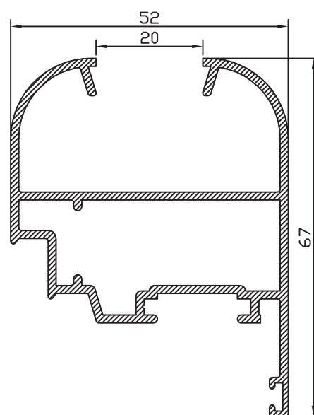
HOJA C/JUNQUILLO C/20 22387
