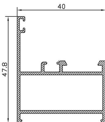
MARCO 28280
