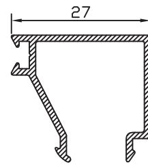
JUNQ. 9.5 22718
