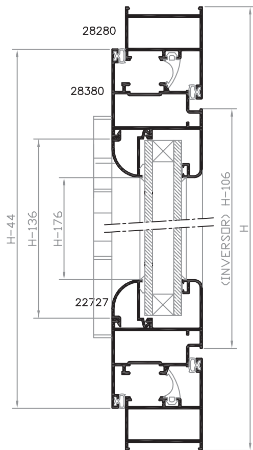
SECCIÓN A-A'
