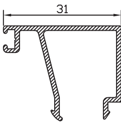
JUNQ. 5.5 22716
