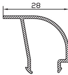
JUNQ. 8.5 22735
