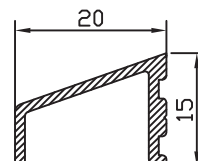
VIERTEAGUAS 22095
