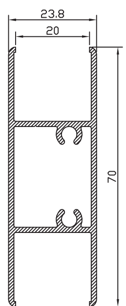
SEPARADOR C/20 28099
