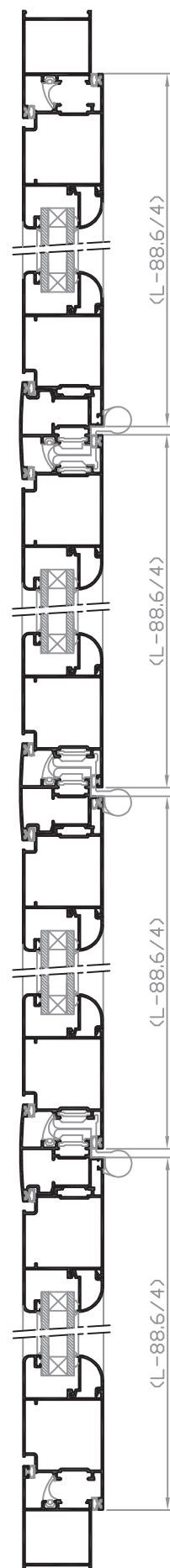
SECCIÓN B-B'
