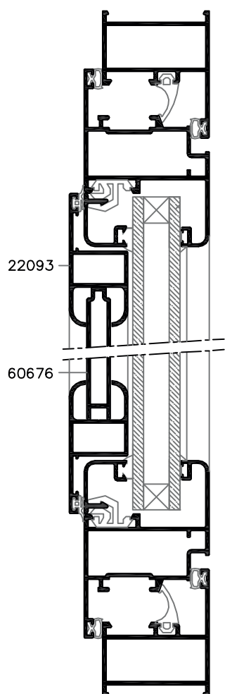
SECCIÓN A-A'
