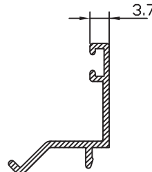
JUNQ. 32.8 22733
