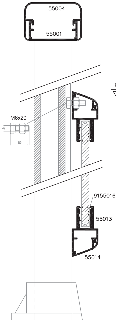
SECCIÓN A-A'
