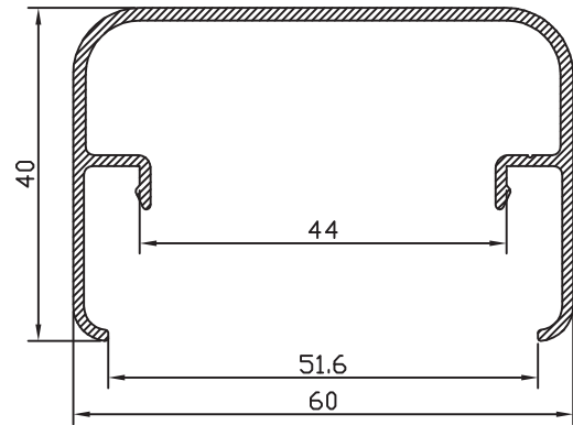
PASAMANOS 60x40 55004
