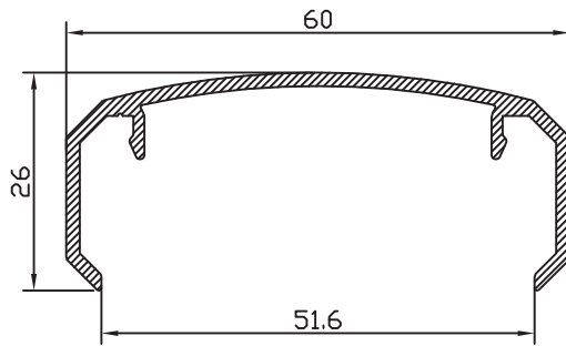
PASAMANOS OCTOGONAL 55018
