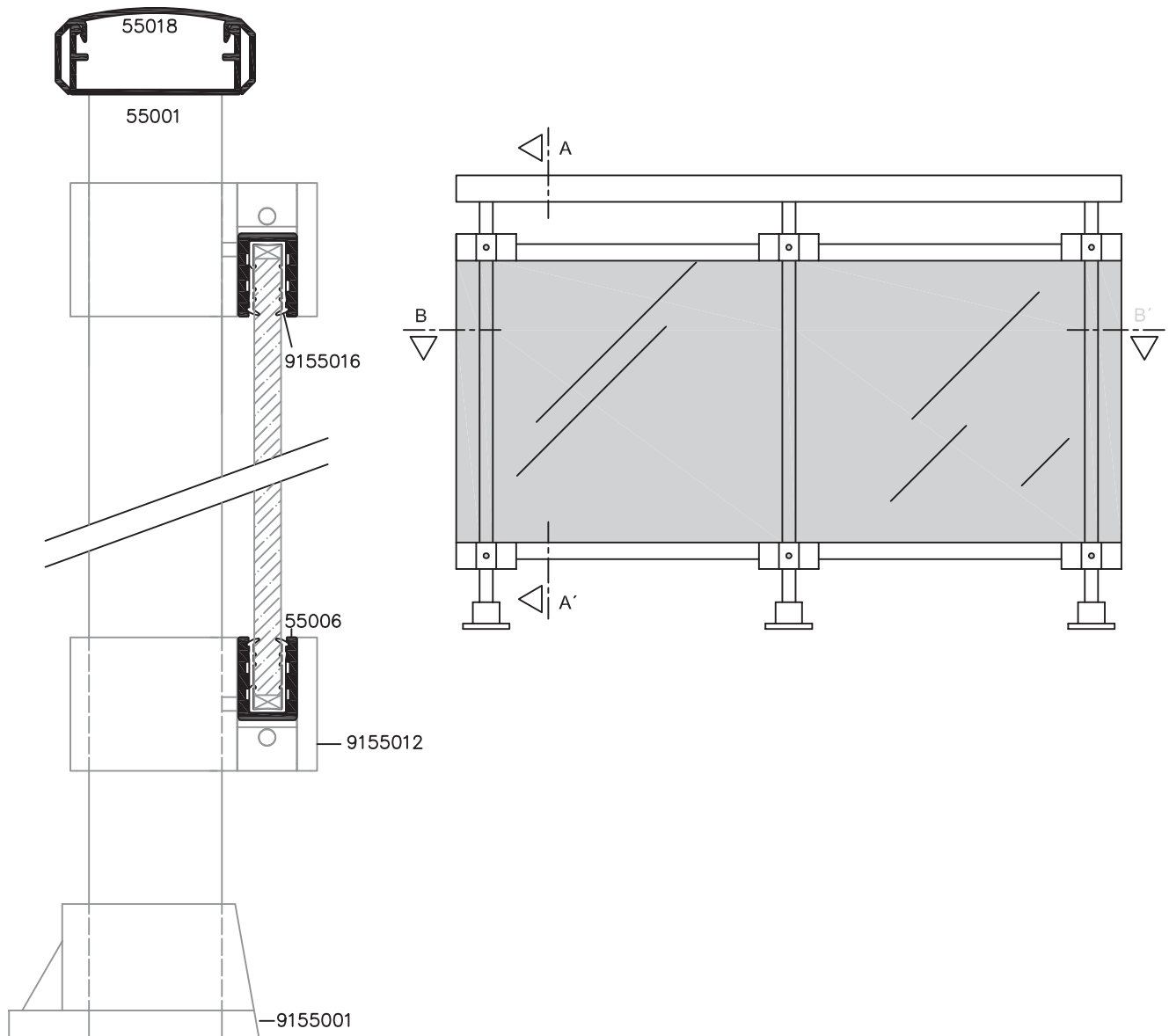
SECCIÓN B-B'
