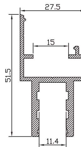
U PORTAVIDRIO 55013
