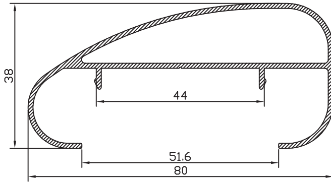
PASAMANOS 80x38 55010
