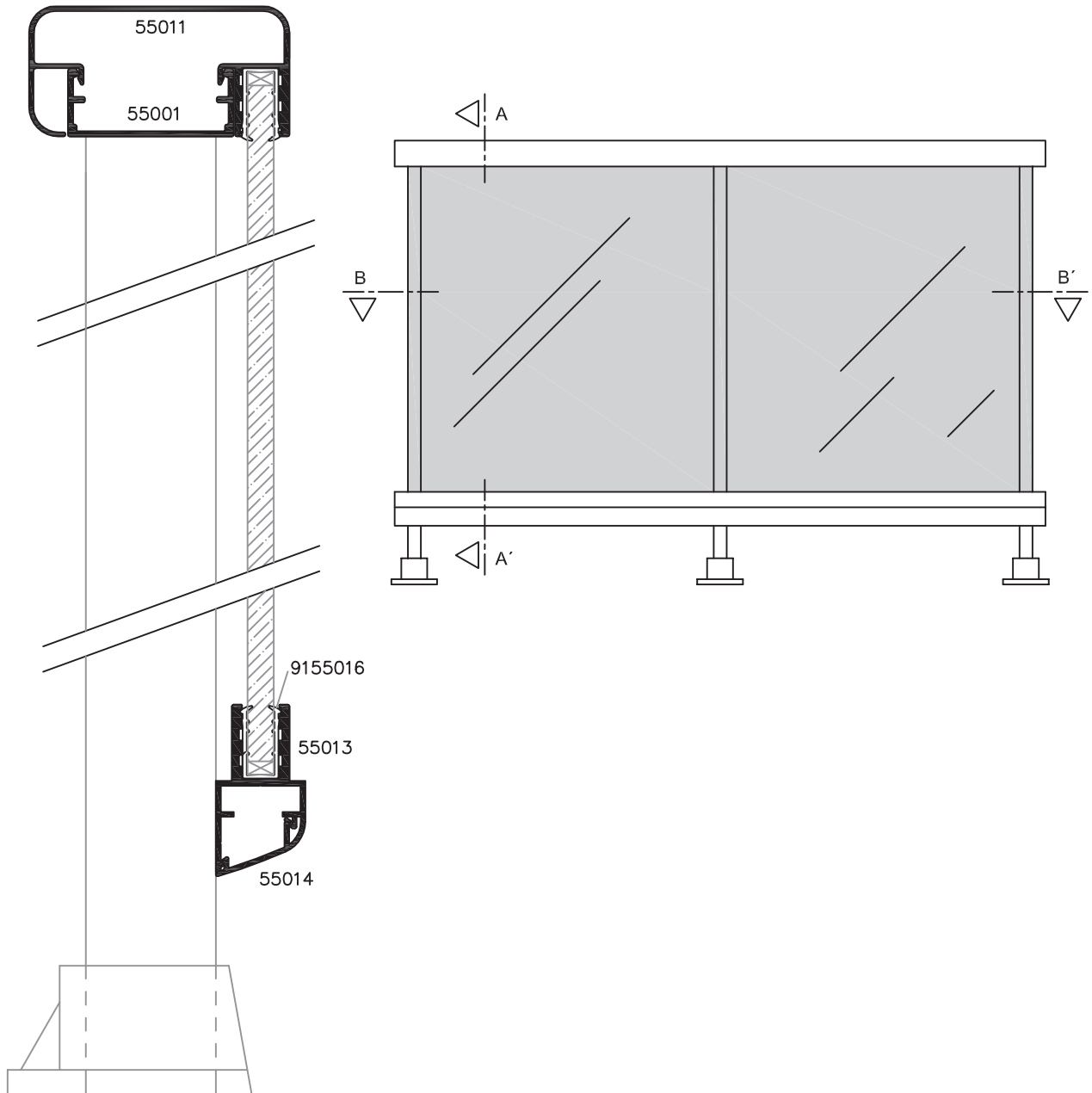
SECCIÓN A-A'
