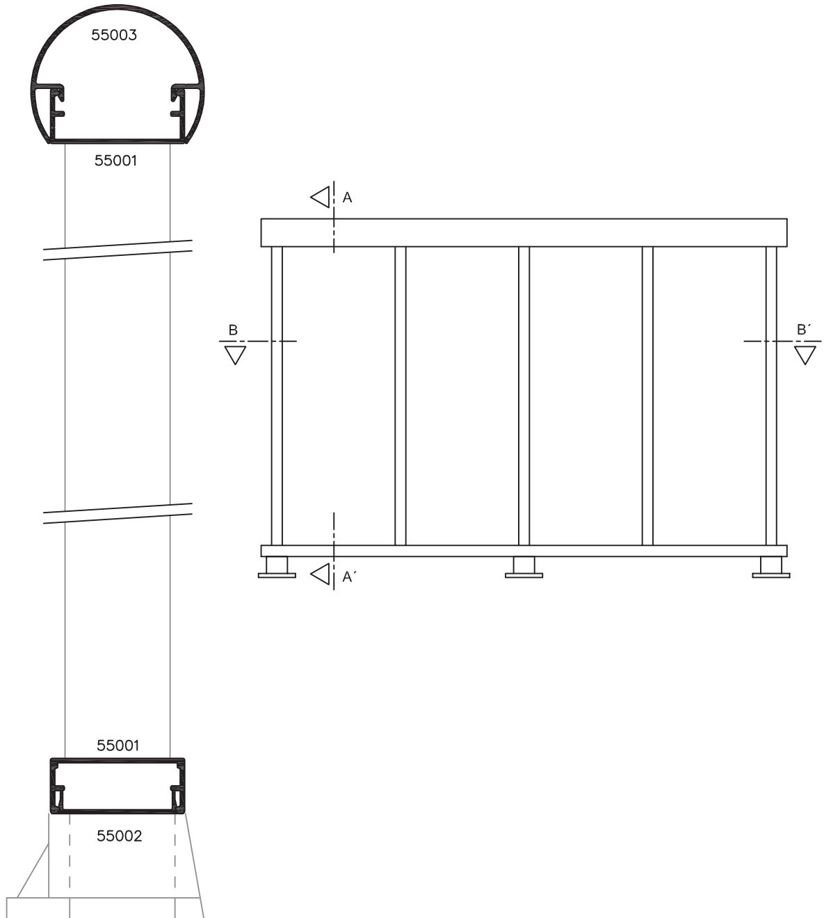
SECCIÓN A-A'
