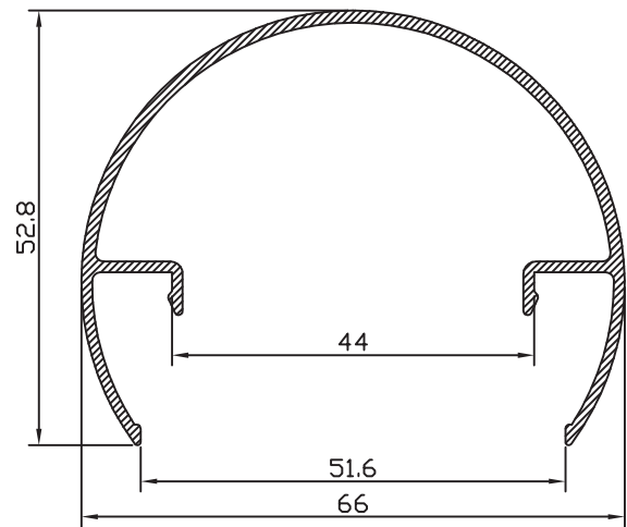
PASAMANOS REDONDO 55003
